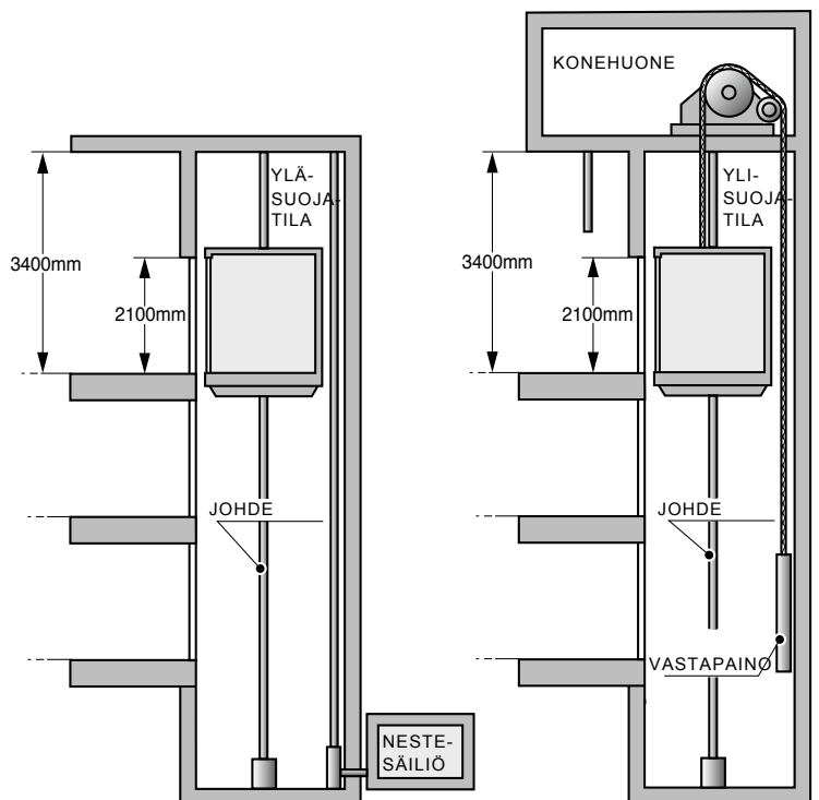
Hydraulinen hissi
