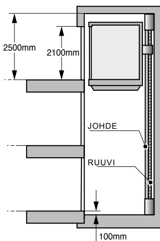
Ruuvikäyttöinen hissi
